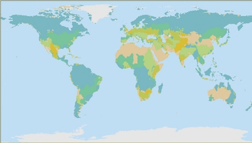
Ressources 2005 en eau des bassins hydrographiques, (bleu, vert, beaucoup ; orange, jaune peu) source : World Resources Institute 2007
